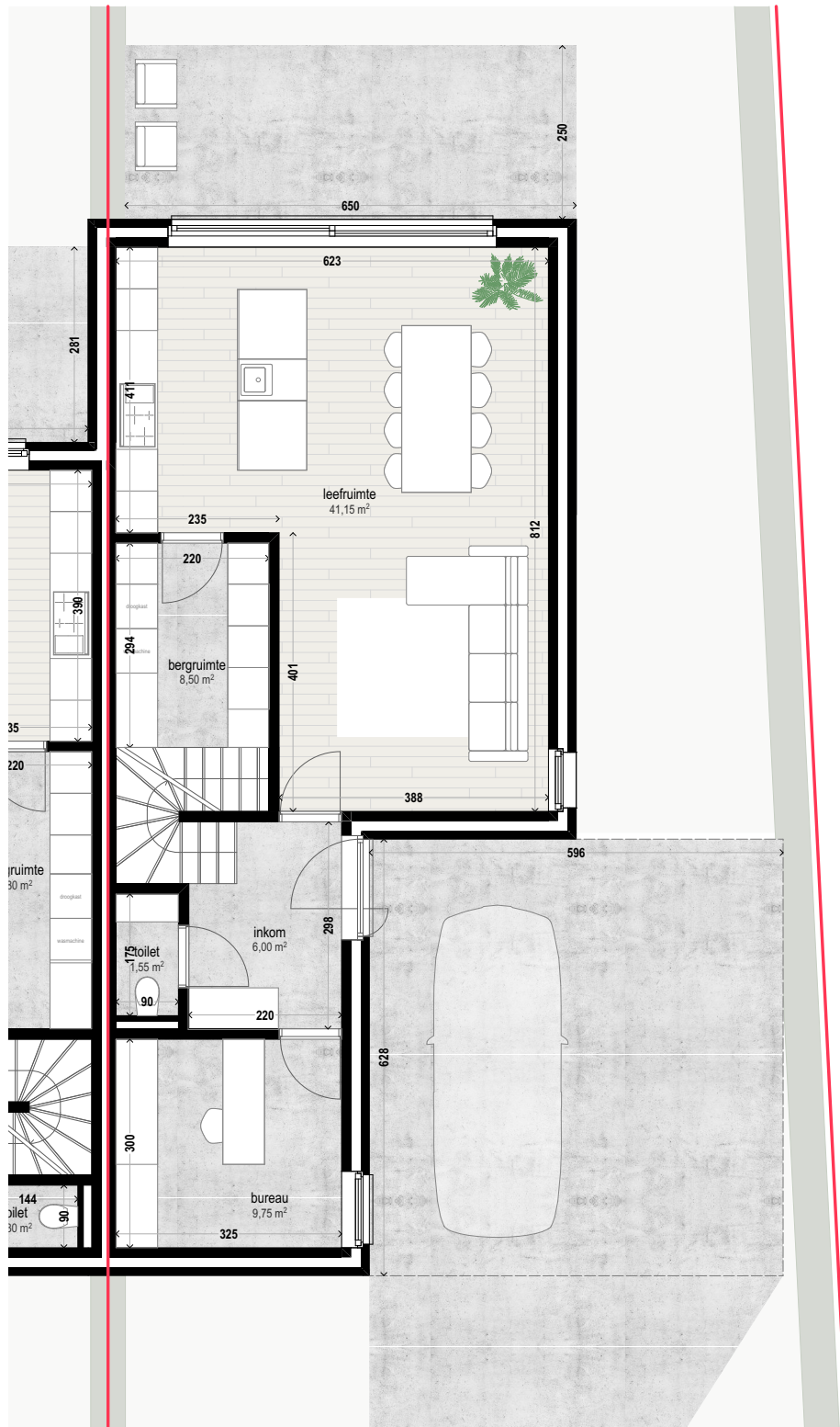
begane grond 85.45 m 2
